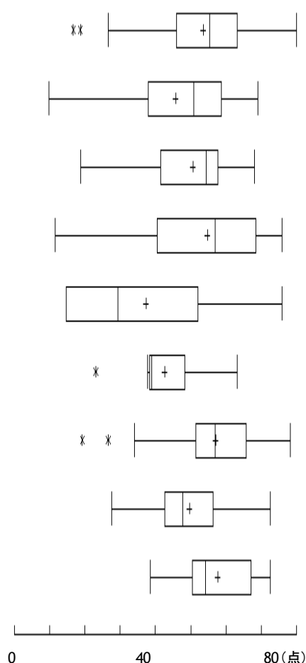
図 1 教科別得点分布の箱ひげ図
