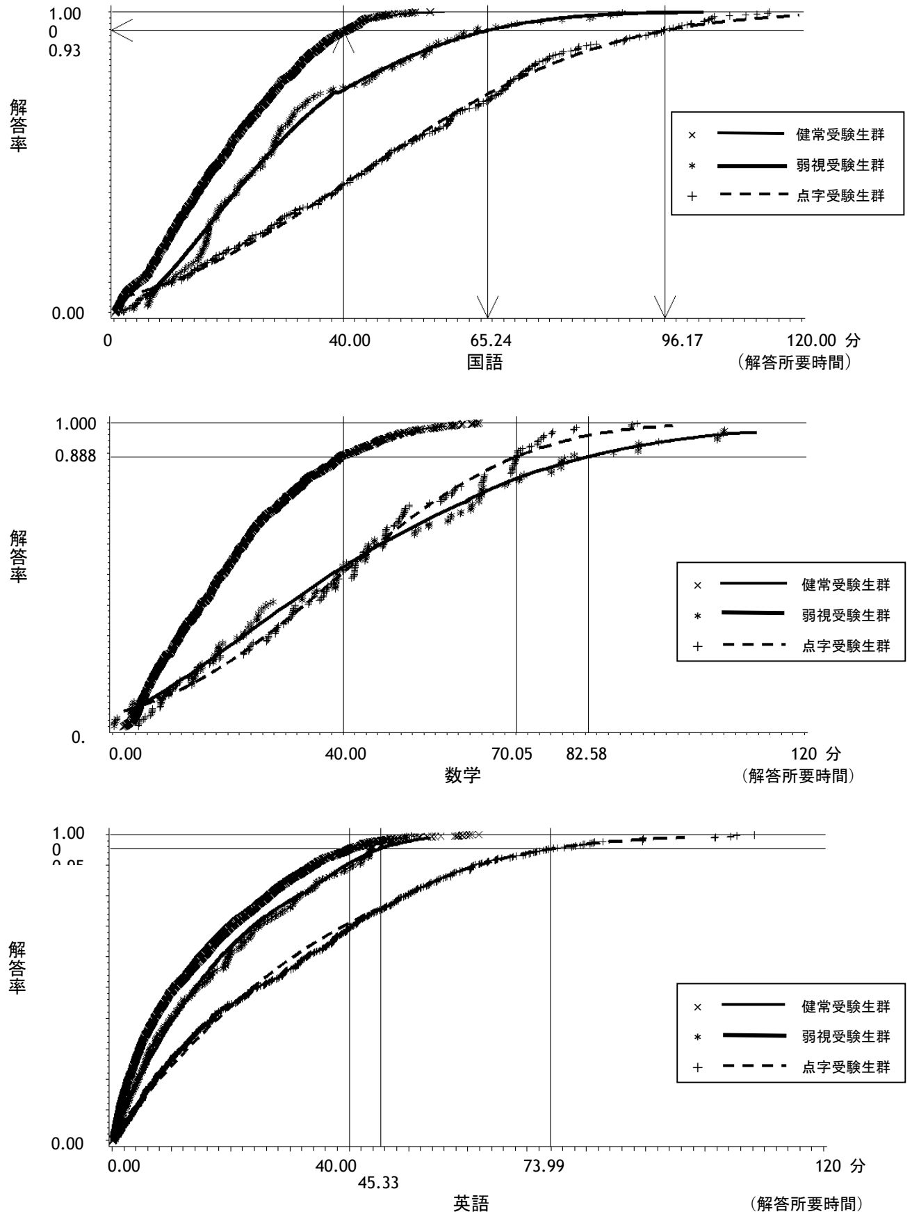
図 3 項目累積型時間－解答率曲線
